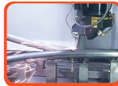
3. 3D lasersnijden
